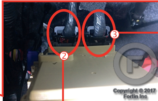
Back of Fuse Box Au dos de la boîte à fusibles
